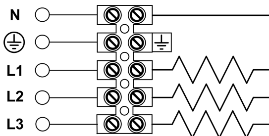
Třífázové připojení
