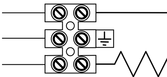
Jednofázové připojení
